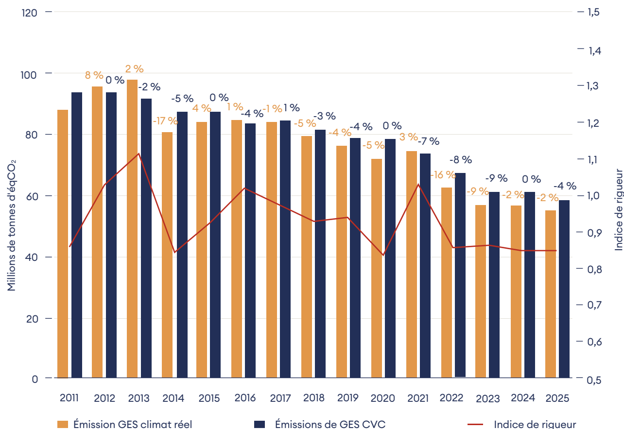
Figure 4.4.1.a – Émissions de GES dans secteur des bâtiments avec et sans correction des variations du climat (CVC)
