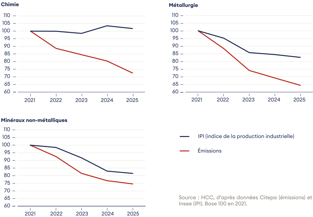
Figure 4.3.1.c – Comparaison entre l'évolution des émissions de GES et l'évolution de la production (IPI) pour les principaux sous-secteurs émetteurs
