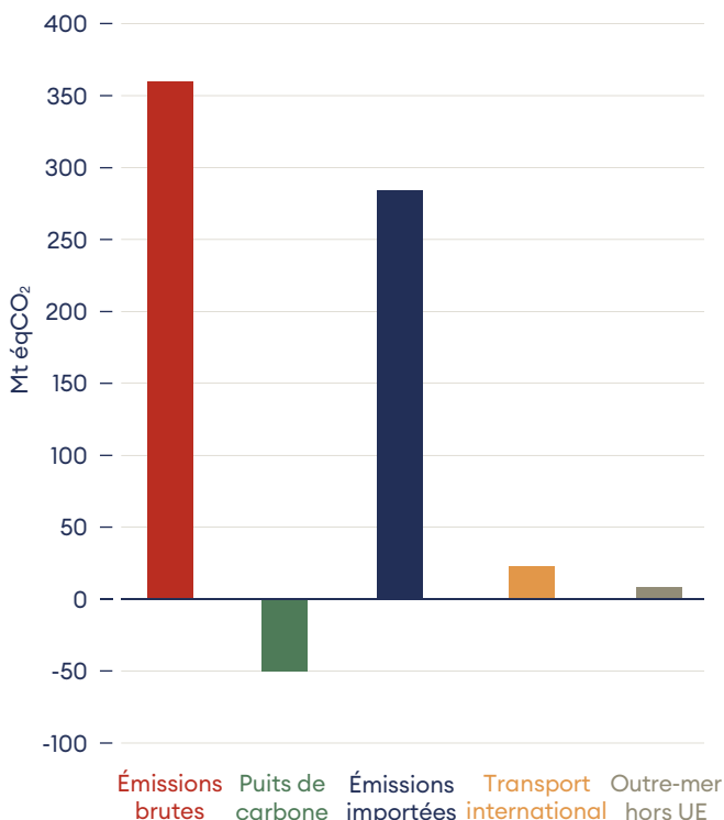
Figure 3.a – Grandes composantes de l'impact climatique de la France
