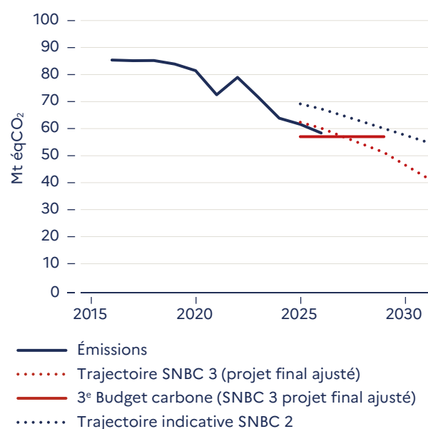
Figure 4.3.1.b – Emissions du secteur de l'industrie depuis 2015, budget carbone et trajectoire indicative du projet de SNBC 3 et trajectoire indicative de la SNBC 2
