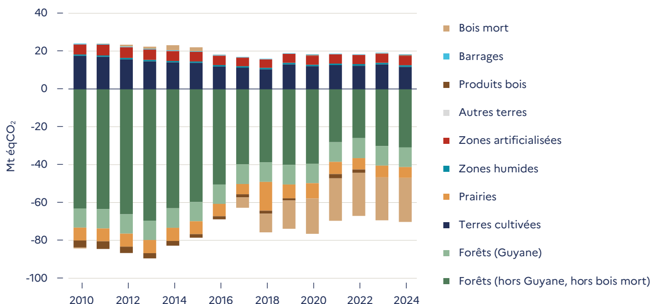
Figure 4.7.1.b – Évolution des composantes du puits de carbone UTCATF national depuis 2010
