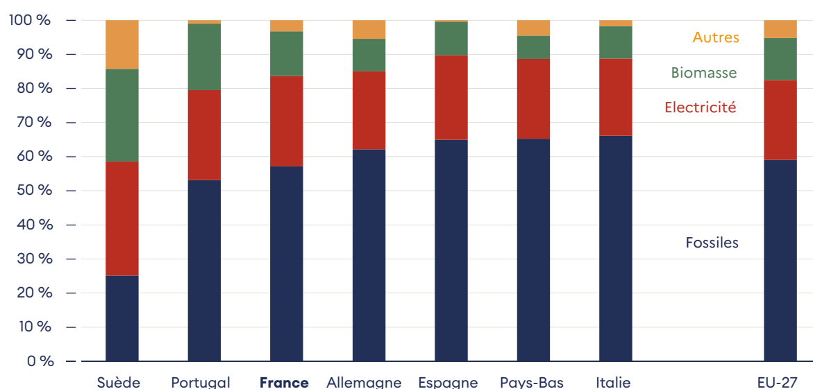
Figure 4.5.2.b – Comparaison de la part de l'électricité dans l'énergie finale consommée dans différents pays en 2024
