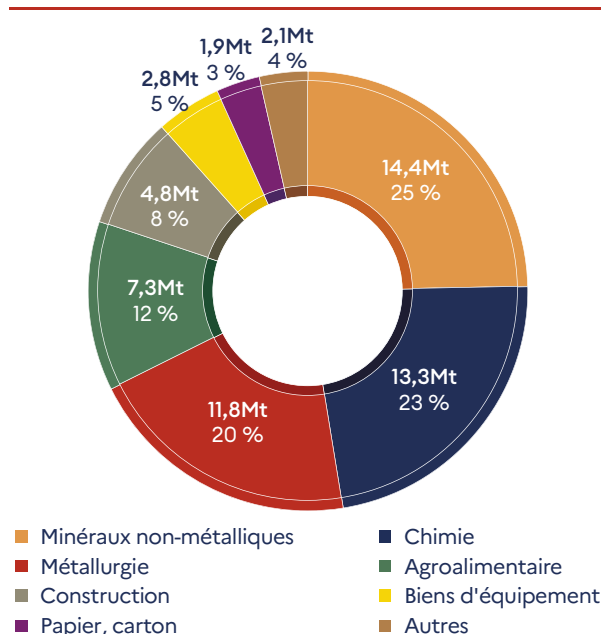
Figure 4.3.1.a – Répartition des émissions par sous-secteur industriel pour l'année 2025
