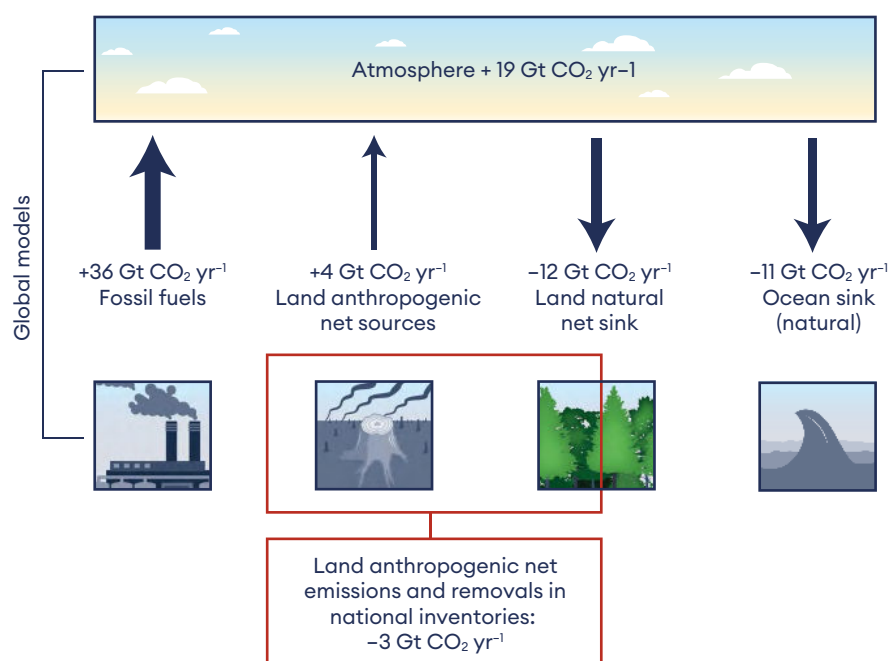
Figure 4.7.1.d – Différences de périmètre d'estimation des flux de CO 2 anthropiques du secteur UTCATF
