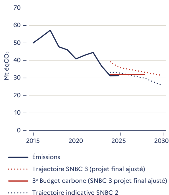
Figure 4.5.1.a – Émissions du secteur de l'énergie depuis 2015, budget carbone et trajectoire indicative du projet de SNBC 3 et trajectoire indicative de la SNBC 2
