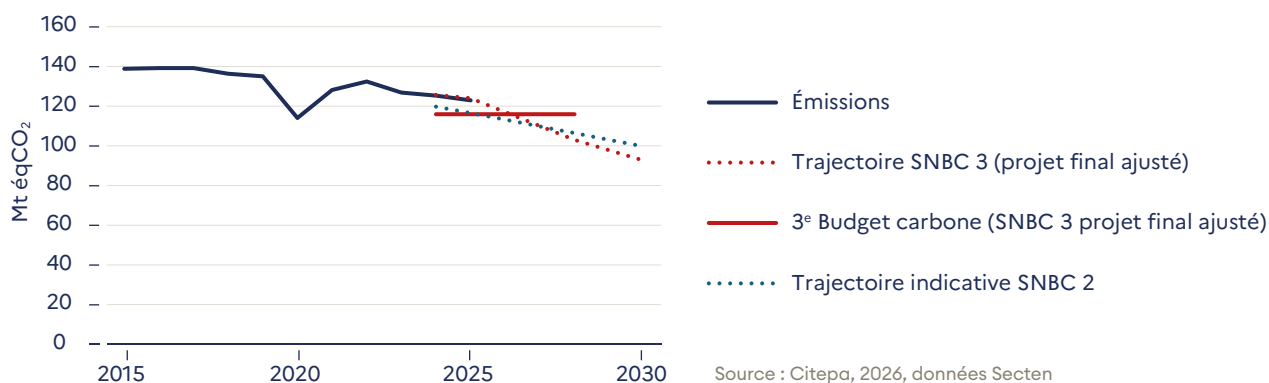
Figure 4.1.a – Émissions du nationales des transports depuis 2015 et trajectoire indicative du projet de SNBC 3
