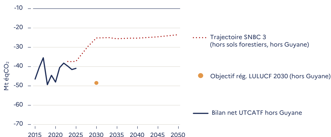
Figure 4.7.1.c – Évolution du puits de carbone UTCATF depuis 2015, trajectoires SNBC 3 et objectif du règlement UE UTCATF
