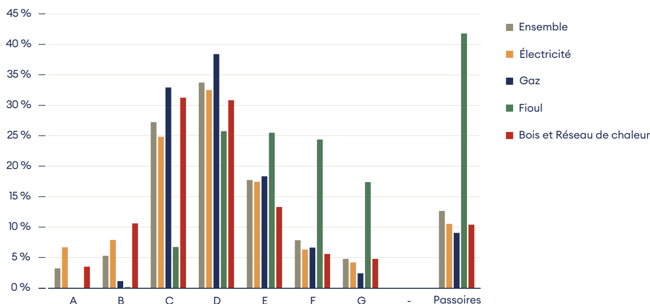
Figure 4.4.3.c – Répartition des sources d'énergie selon le DPE
